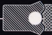
Polypak/Pip Ring Combination
